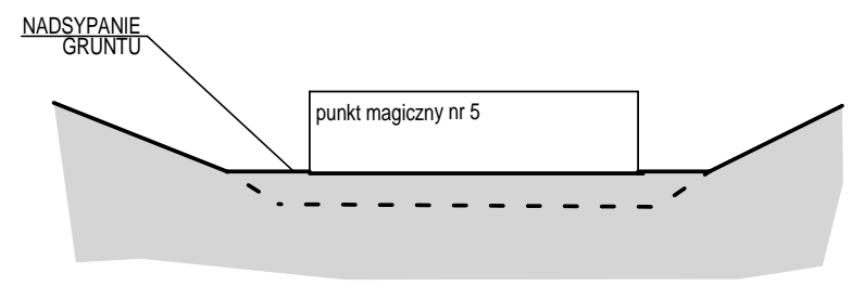
SCHEMAT FUNDAMENTY KAMIENNE NA GŁ. 5,50m
